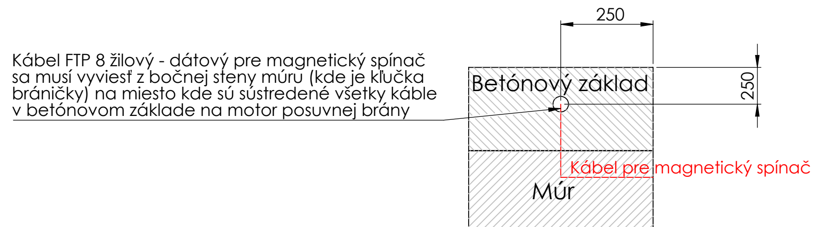
Pohľad zvrchu na betónový základ a múr
